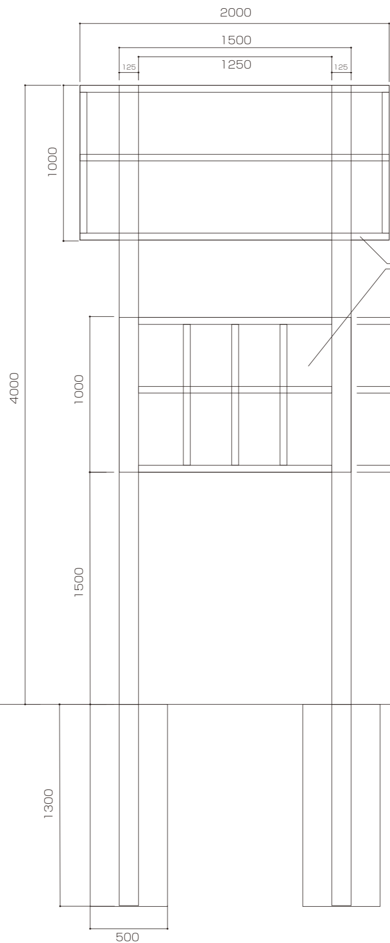
正面構造
